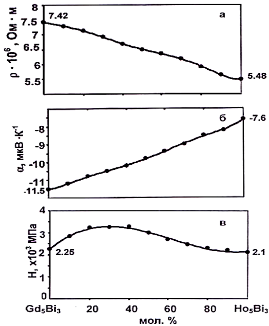
Рисунок 2 – Концентрационные зависимости удельного электросопротивления (а), термо-э.д.с.(б) и микротвердости (в) твердых растворов Gd_{5-x}Ho_xBi_3 ; ( x = 0.5 \div 4.5 ) при 298 К
